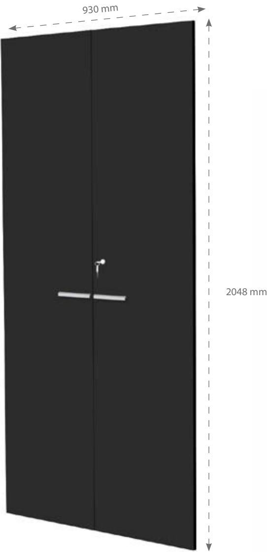
G340022-NP-T2 / 930x19x2048
